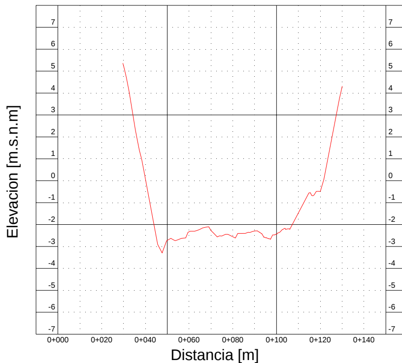
Figura B 2-7: Sección Transversal K44+775
