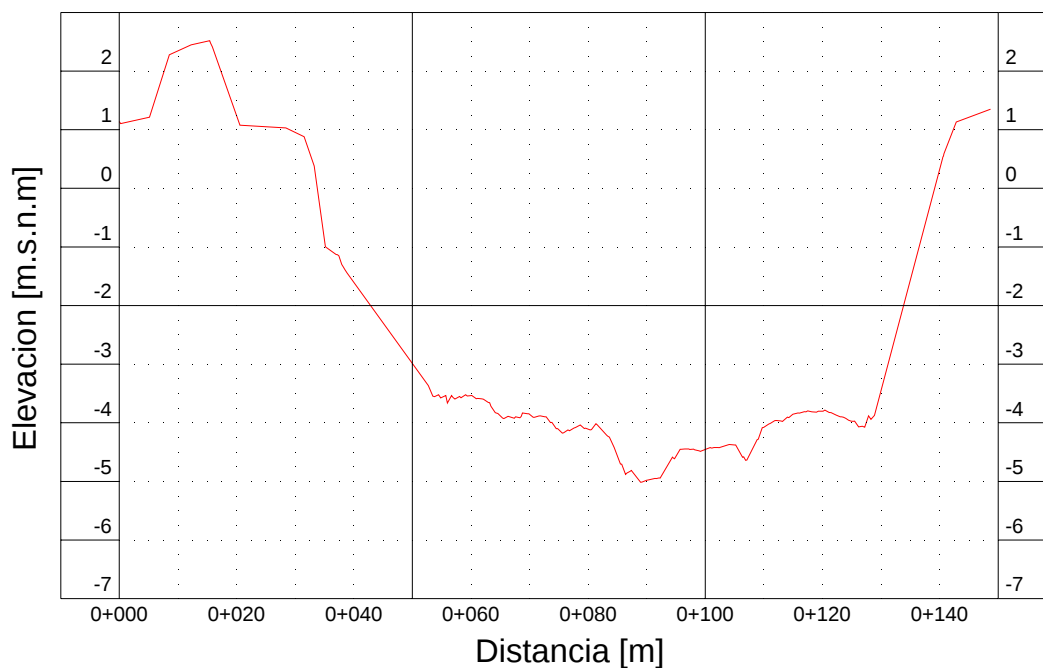
Figura B 2-15: Sección Transversal K92+375
