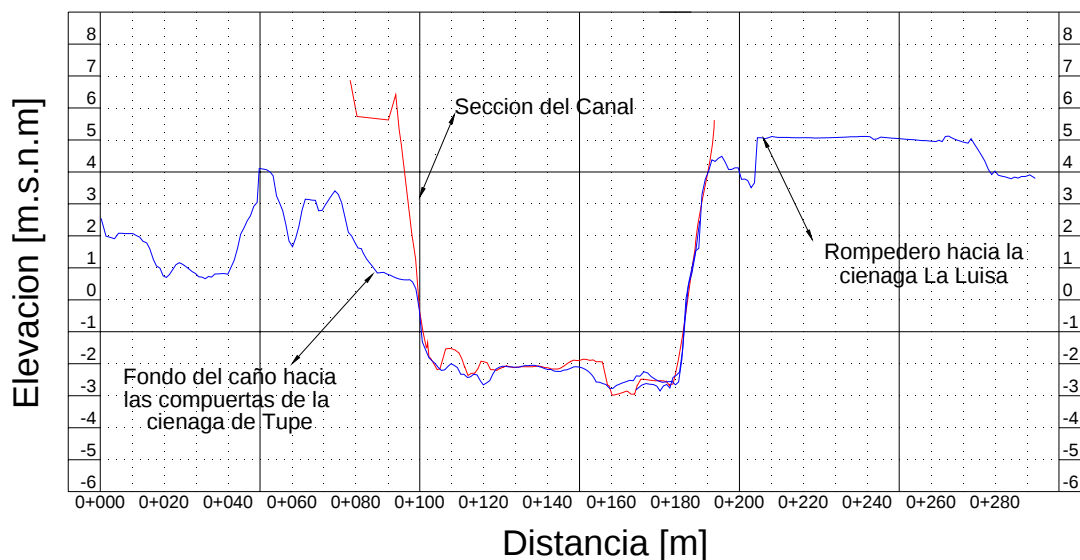
Figura B 2-7: Sección Transversal K44+775
