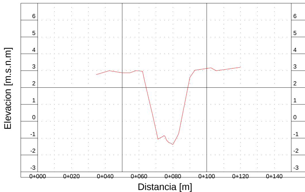
Figura B 2-16: Sección Transversal K0+310 Correa
