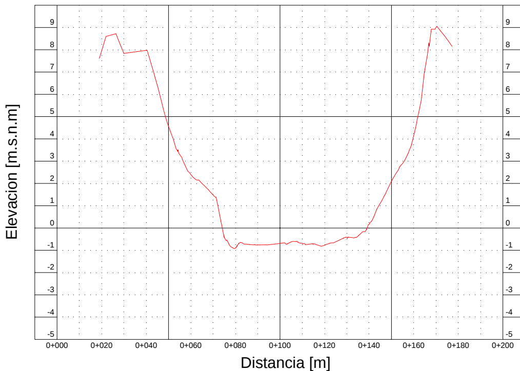
Figura B 2-4: Sección Transversal K19+635
