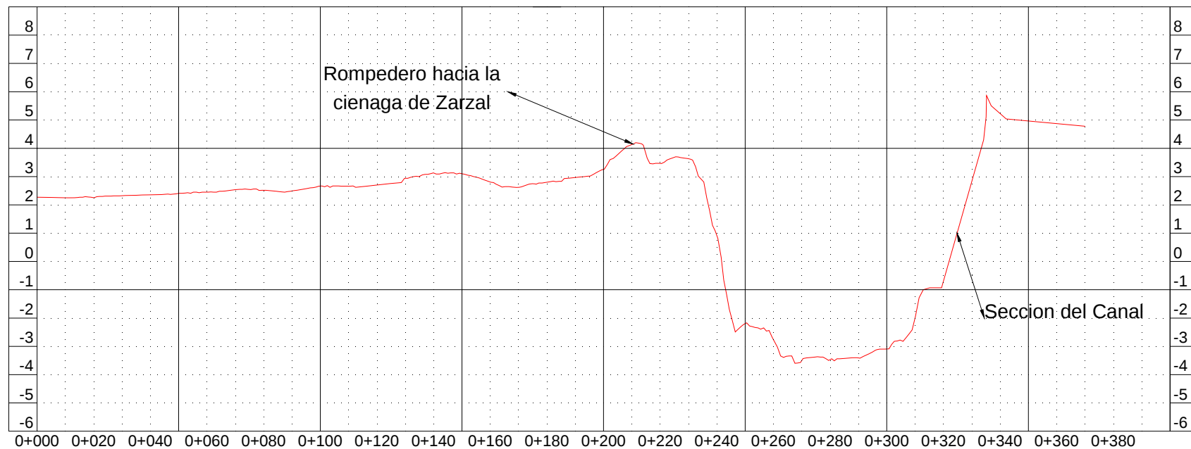
Figura B 2-9: Sección Transversal K48+596
