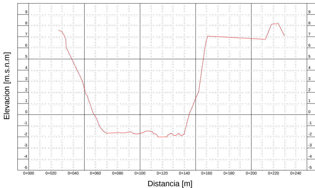
Figura B 2-4: Sección Transversal K19+635
