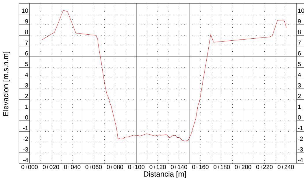
Figura B 2-2: Sección Transversal K6+413
