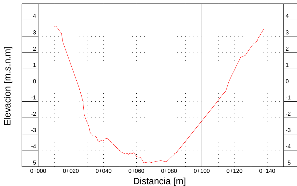
Figura B 2-13: Sección Transversal K83+976
