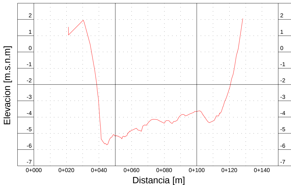
Figura B 2-15: Sección Transversal K92+375
