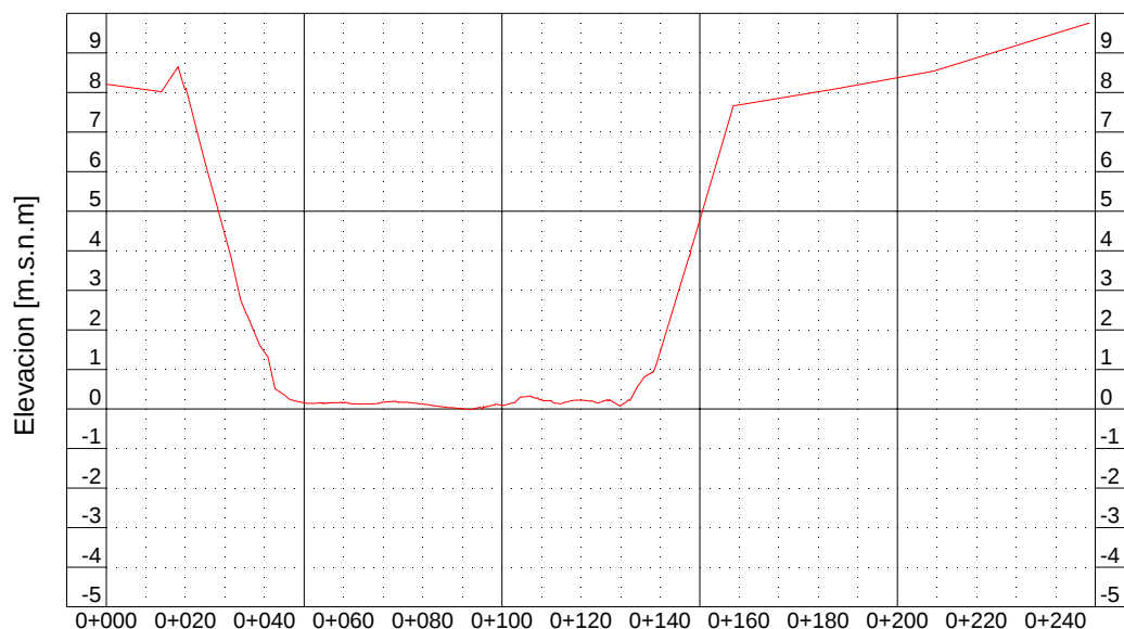
Figura B 2-1: Sección Transversal K0+675
