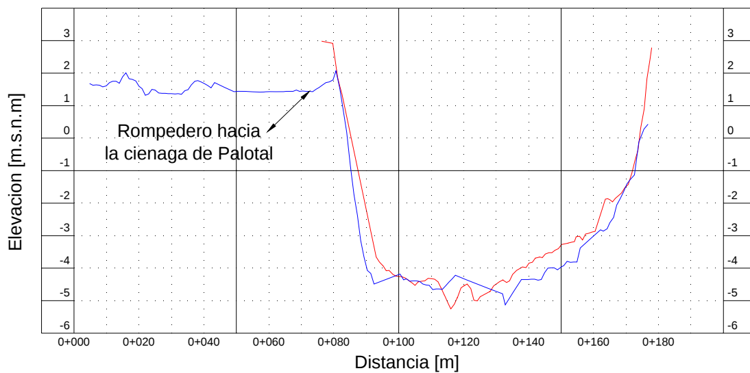
Figura B 2-13: Sección Transversal K83+976
