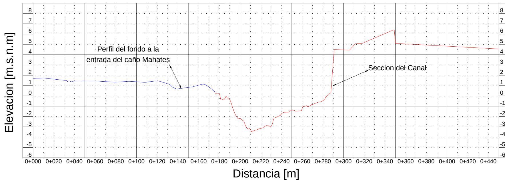
Figura B 2-10: Sección Transversal K52+000
