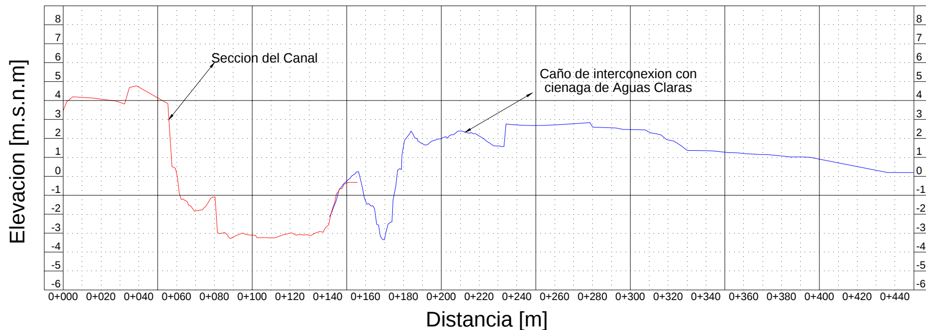
Figura B 2-11: Sección Transversal K64+913
