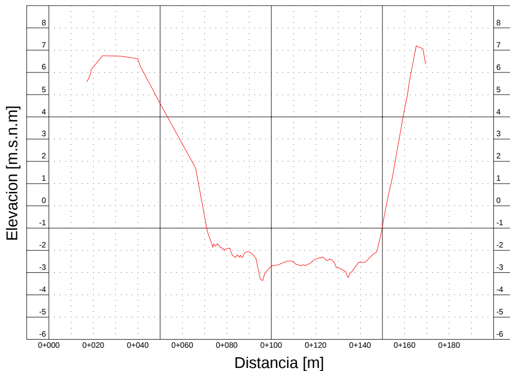
Fotografía B 2-1: Comisión topobatimetrica Figura B 2-5: Sección Transversal K38+000
